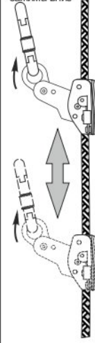
Рис. 6. Движение зажима вниз
