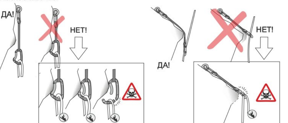
Рис. 6. Установка оттяжек
