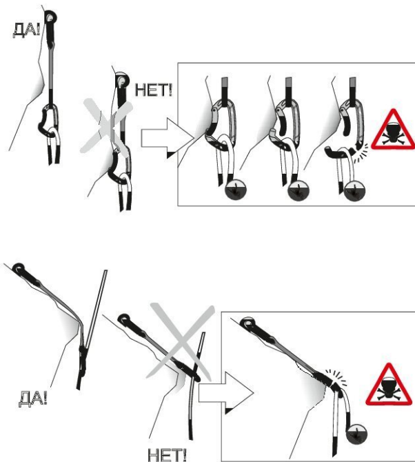
Рис. 4. Установка оттяжек
