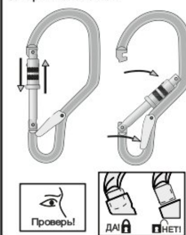
Рис. 3. Открытие/ закрытие/ фиксация запорных элементов
